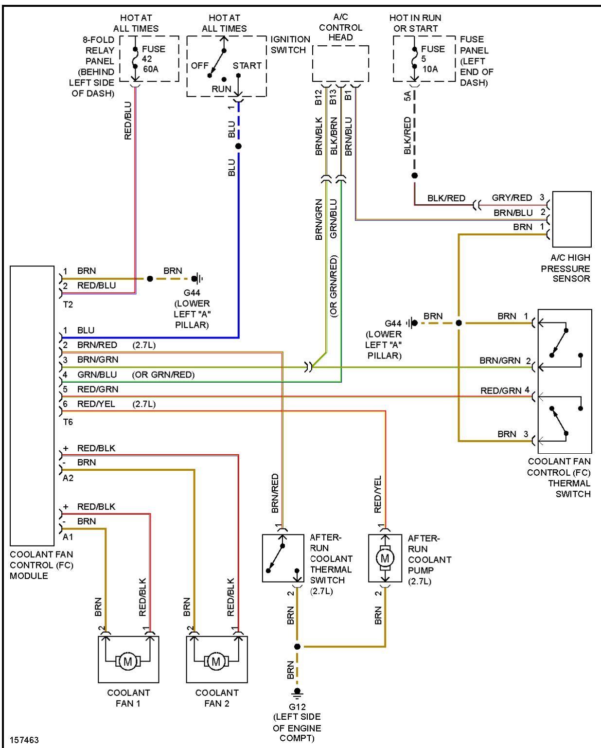
Fig. 10: 2.7L Turbo, Cooling Fan Circuit
